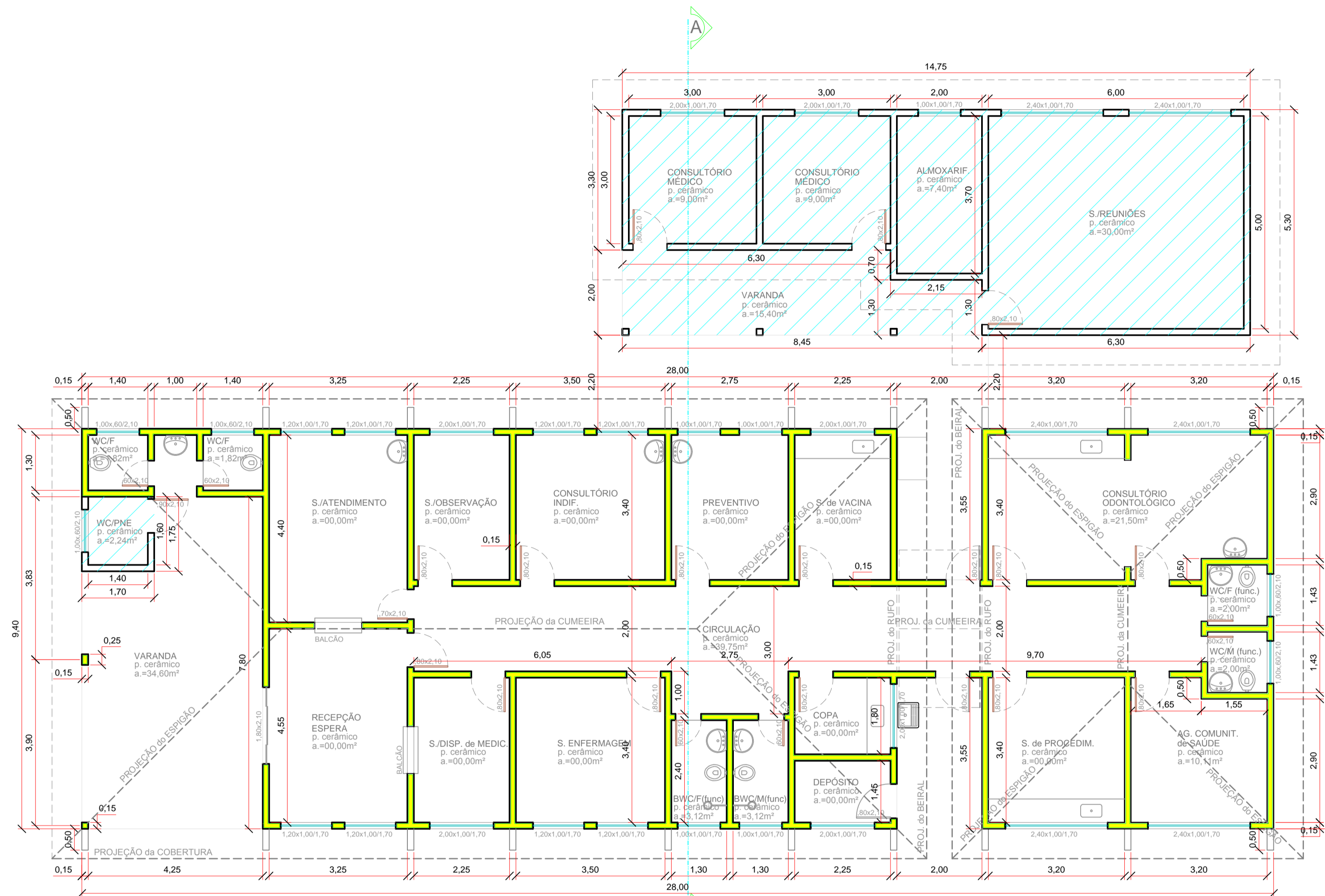
PLANTA BAIXA ESCALA 1/100 █ EXISTENTE A = 249,00 m 2 █ A AMPLIAR A = 78,18 m 2
